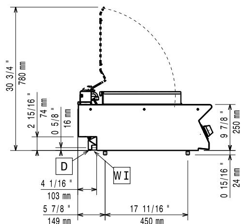
Oldalnézet
